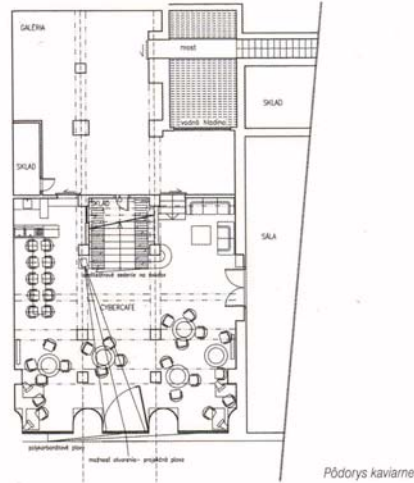
Pôdorys kaviarne
